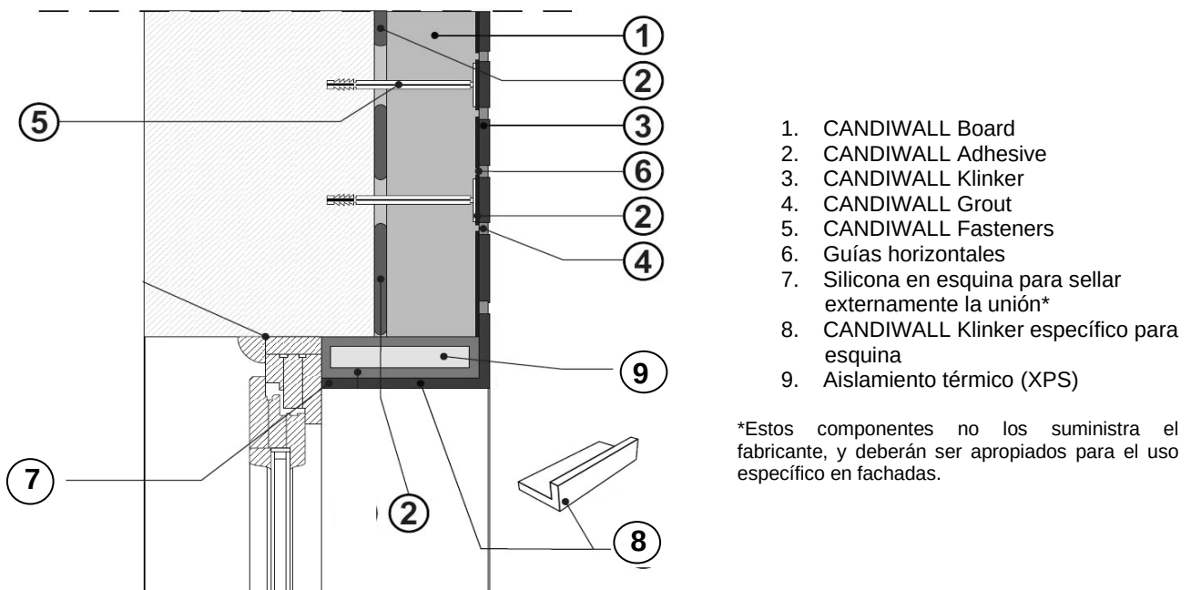
Figura 2. Detalle del sistema CANDIWALL en puertas y huecos
