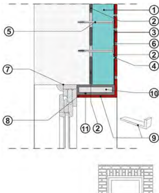
Figura II.5 – Remate com ombreiras de portas e janelas
