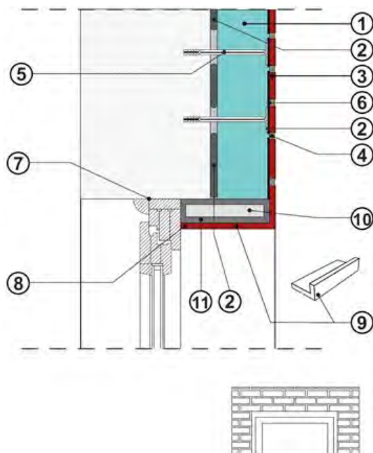
Figura II.4 – Remate com ombreiras de portas e janelas
